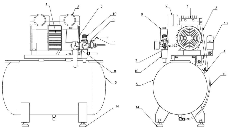
Рисунок 1 Складальне креслення компресора
